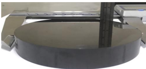
4" SiC 晶錠
